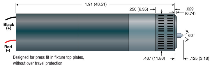
BMP-1-S
