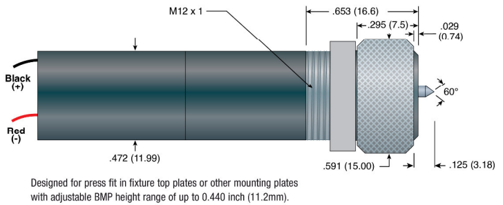
BMP-3
